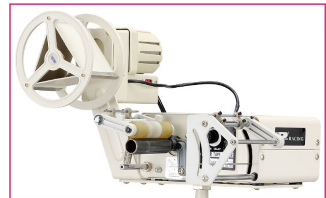
TFU 16-3 / UT-2 上送型送料機(附電動型防止打結裝置)，送料寬度70mm Upper tape feeder (with untangling motor device). Feed width 70mm TFU 16-8 上送型送料機，送料寬度 200mm Upper tape feeder, Feed width 200mm
