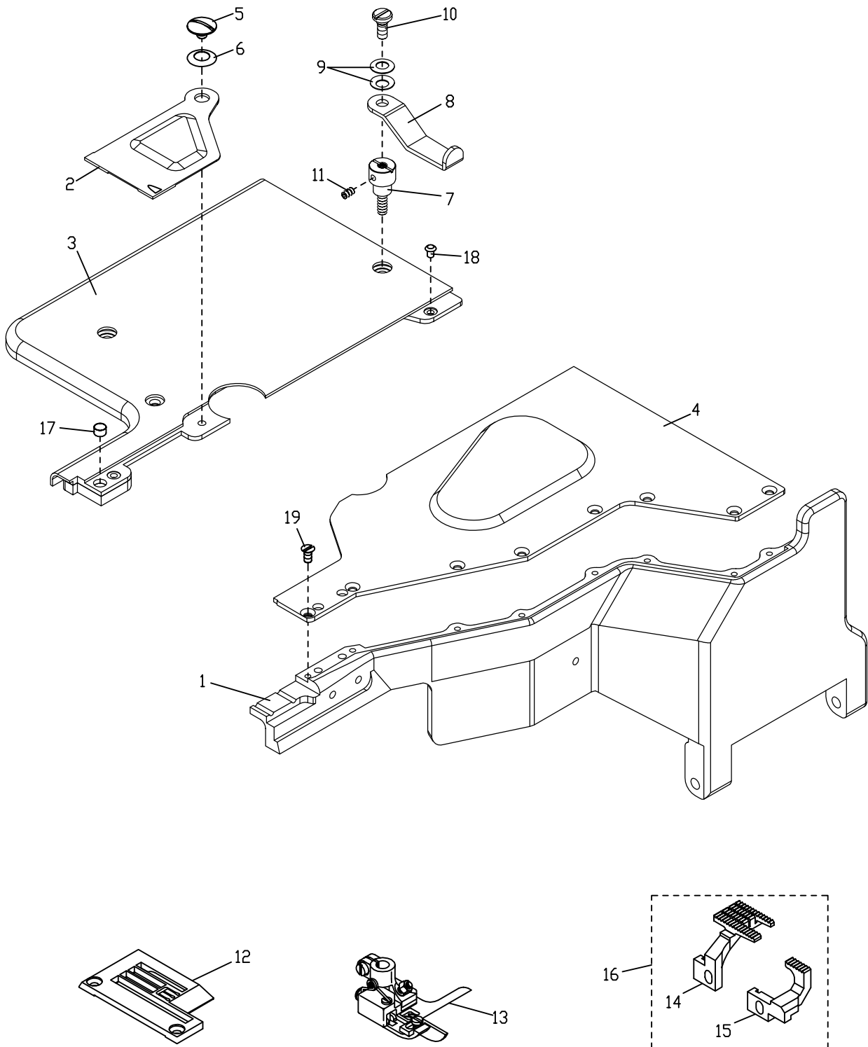
12. 針板編號列表 Needle Plate
