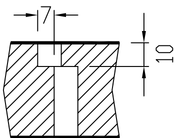
A-A 剖面 A-A SIDE VIEW
