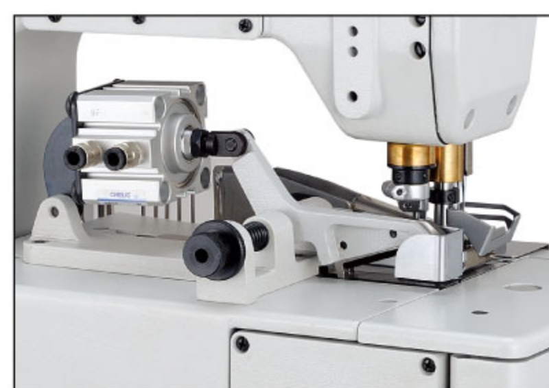
切帶裝置 Tape Cutter TC / TCS
