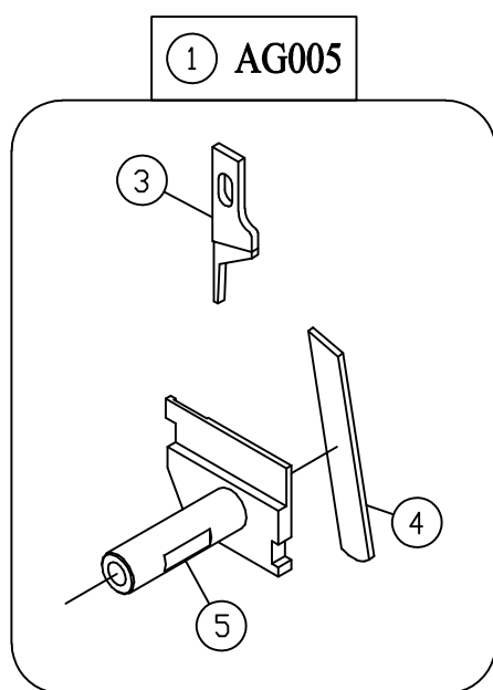
AG005 平寬刀組 3、4 線用
