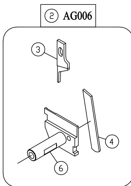
AG006 平寬刀組 5 線用
