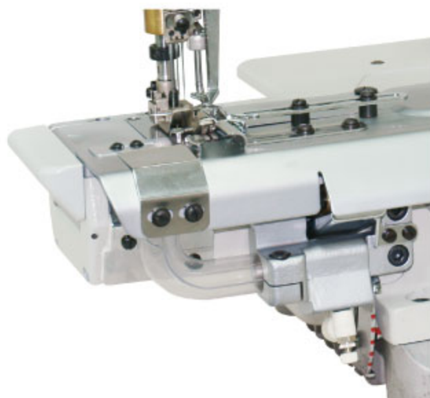
CT9311 / CTD9311
