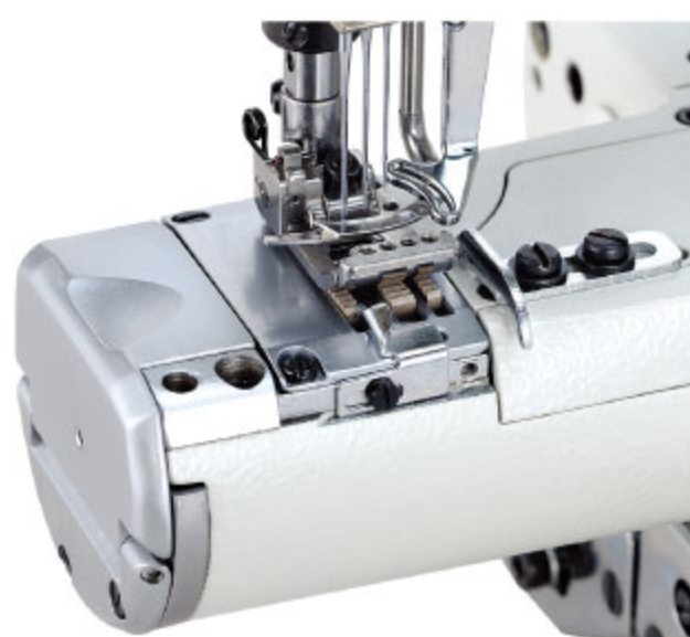
CTD9711(180mm)
