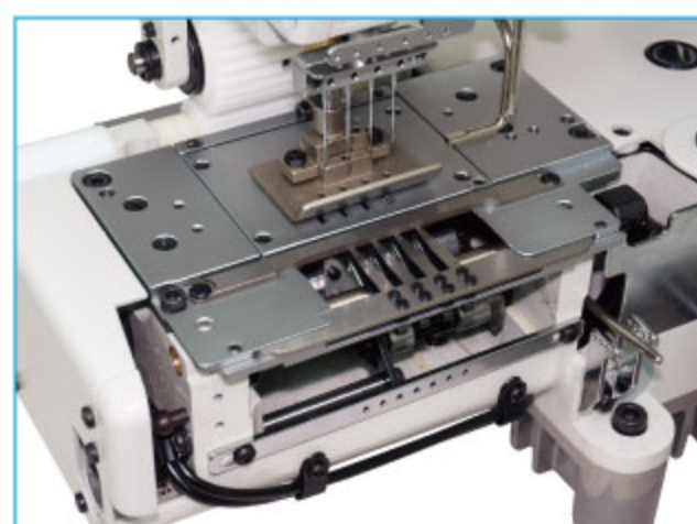
UT04A:切線刀組 Thread trimmer set
