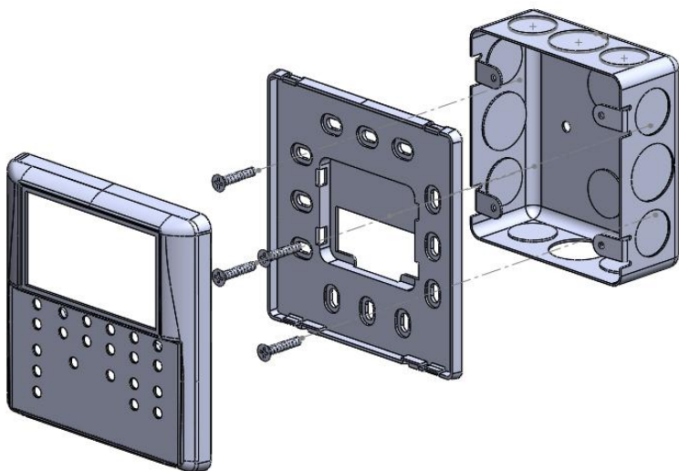
2P 埋入式插座盒 安裝示意圖
