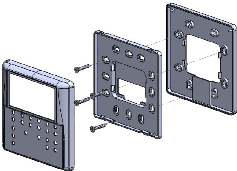
貼壁式 示意圖
